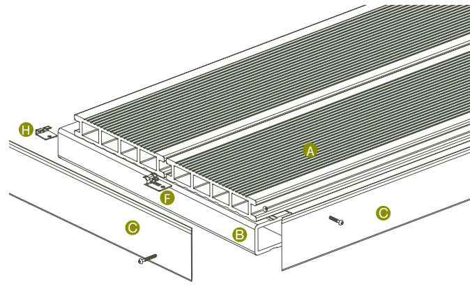
deska komorowa DFDE 162** o strukturze drewna
